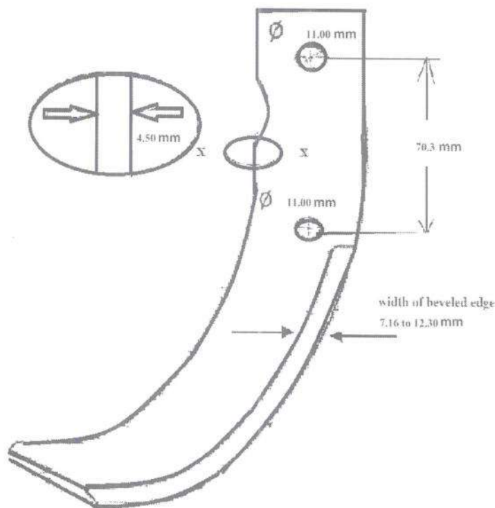
FIG. 3 : ROTOR BLADE
